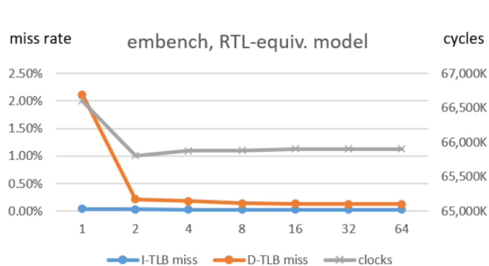
TLB way数とTLBミス率・実行サイクル数
